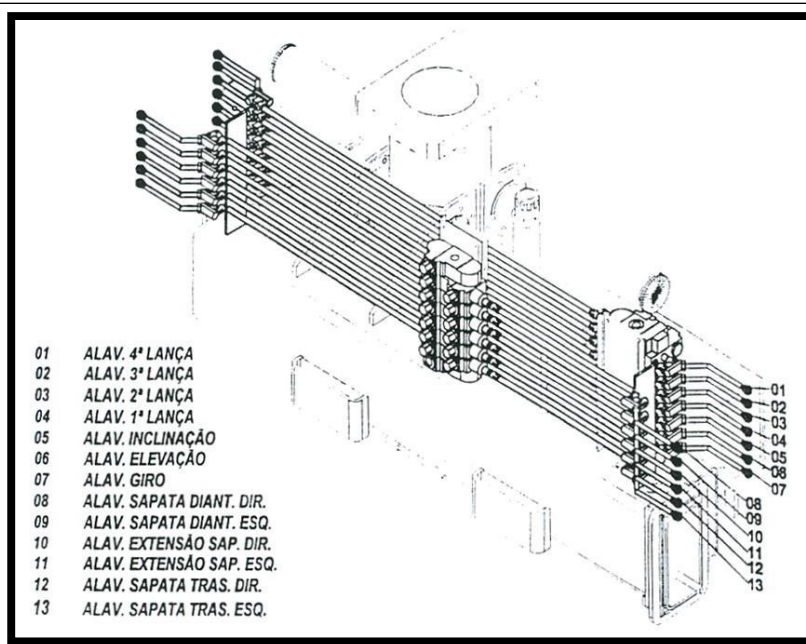
Figura 2 – Alavancas de Comando com acionamento em ambos lados do veículo.
